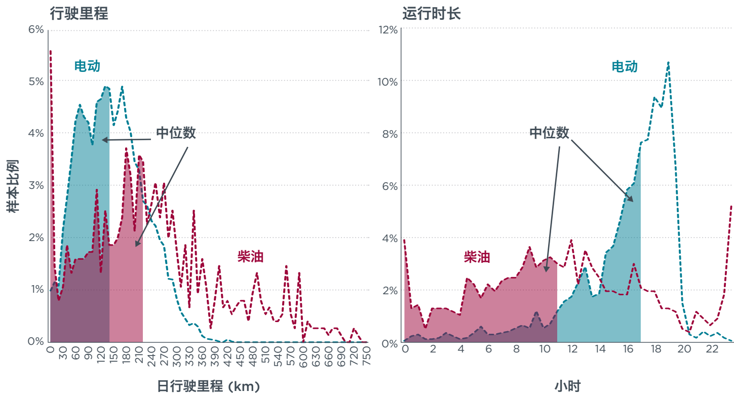
图 3. 电动和柴油半挂牵引车的日行驶里程（左侧，数据精确至10km）和运营时长（右侧），其中实色填充部分代表中位数。
