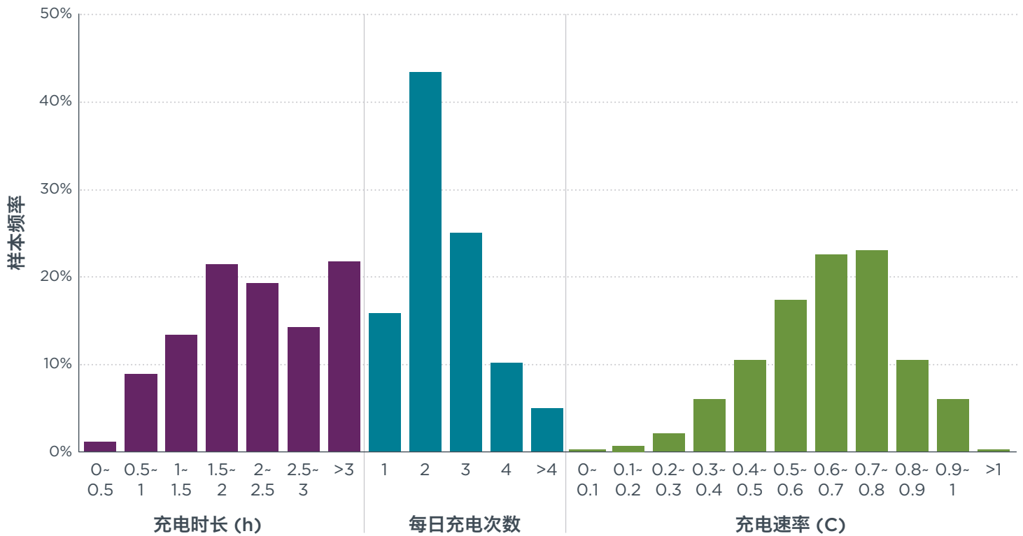
图 4. 本次研究中电动半挂牵引车的充电模式
