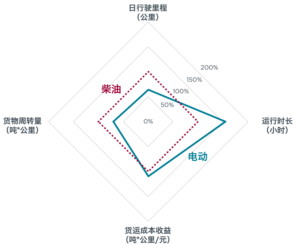
图5. 电动半挂牵引车与柴油车型的运输能力对比
